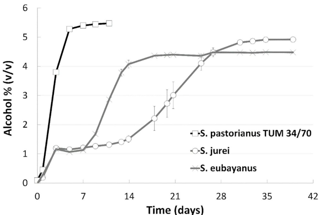
Abbildung 1: Gärungsdiagramm zwischen TUM 34/70, TUM 629 und S. eubayanus (aus [2])
